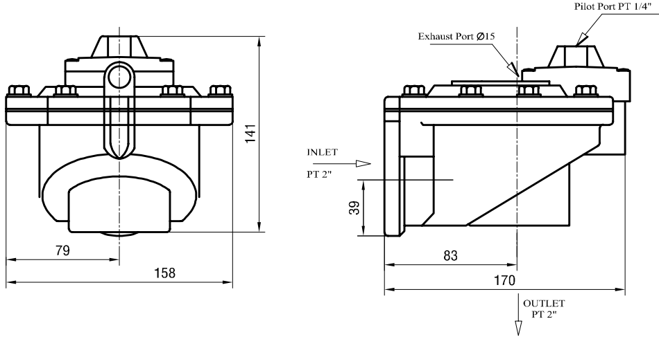
Şekil 13: Uzaktan Kontrol Patlaç Valf Bobinsiz G1 1/2", G2", G2 1/2", G3" Ölçü
