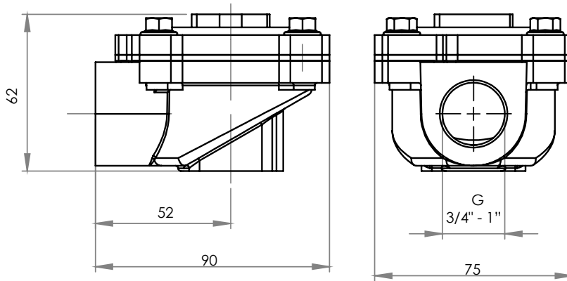
Figure 12: Bobinsiz G3/4", G1" Ölçü Standart Patlaç Valf
