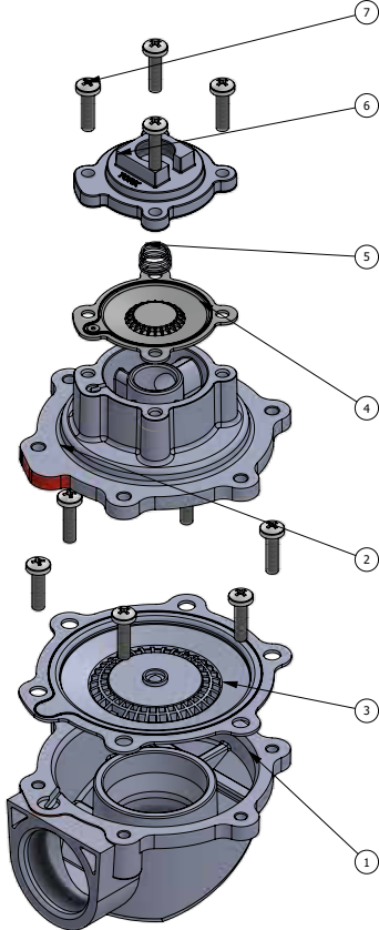
Şekil 5: Uzaktan Kontrol Patlaç Valf Bobinsiz G1 1/2", G2" G2 1/2", G3"
