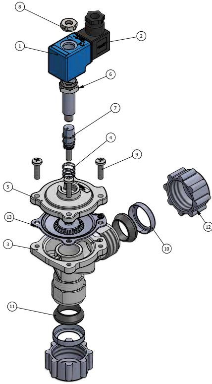
Şekil 6: Rakor Bağlantılı Patlaç Valf Bobinli G ¾"-G3/4", G1"-G1"
