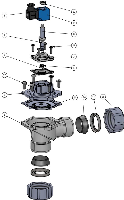
Şekil 7: Rakor Bağlantılı Patlaç Valf Bobinli G 1½" - G 1½"
