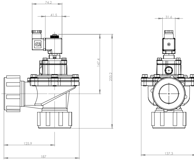
Figure 14: Rakorlu Patlaç Valf Bobinli G3/4", G1", G1 1/2" Ölçü
