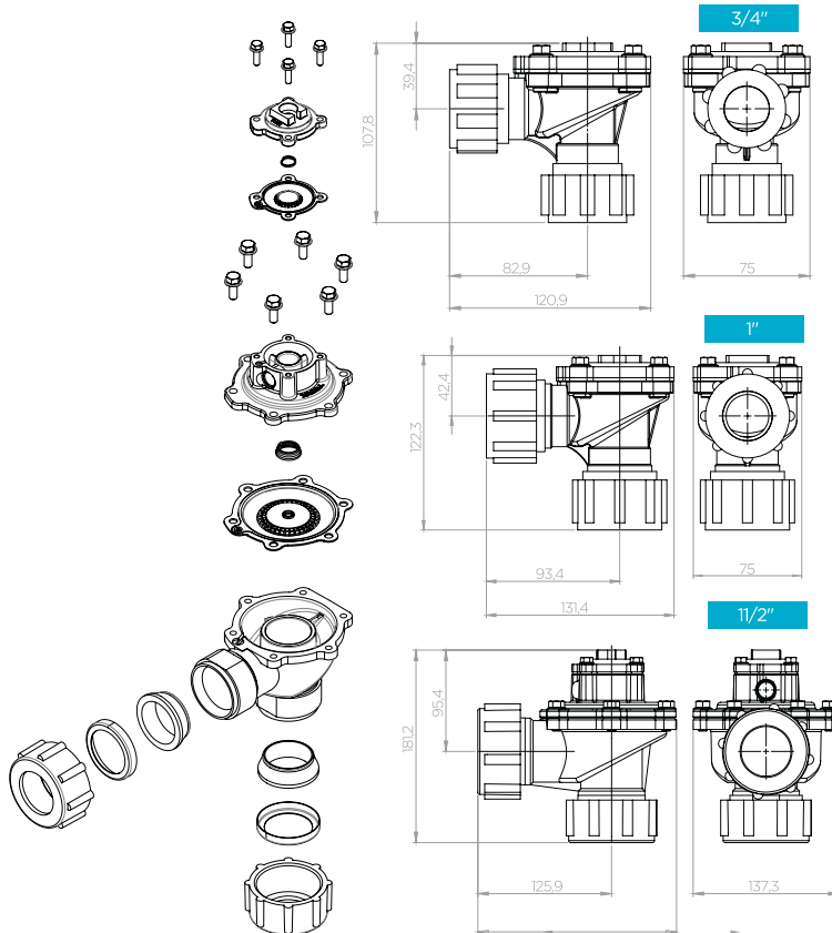
Figure 15: Rakorlu Yüksek Basınç Patlaç Valf Bobinli G1 1/2" Ölçü
