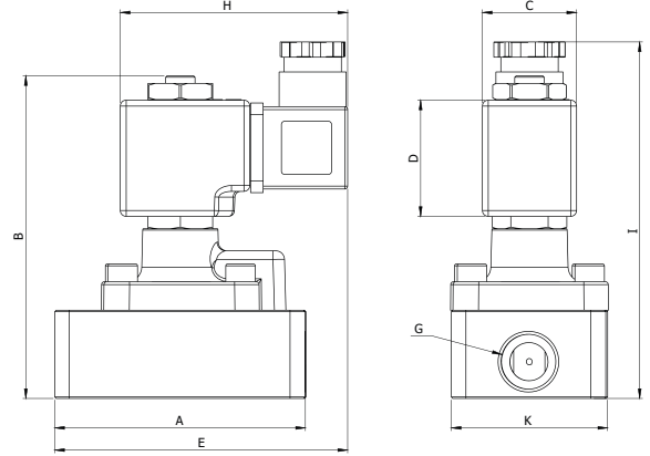
Ölçüler (mm)
