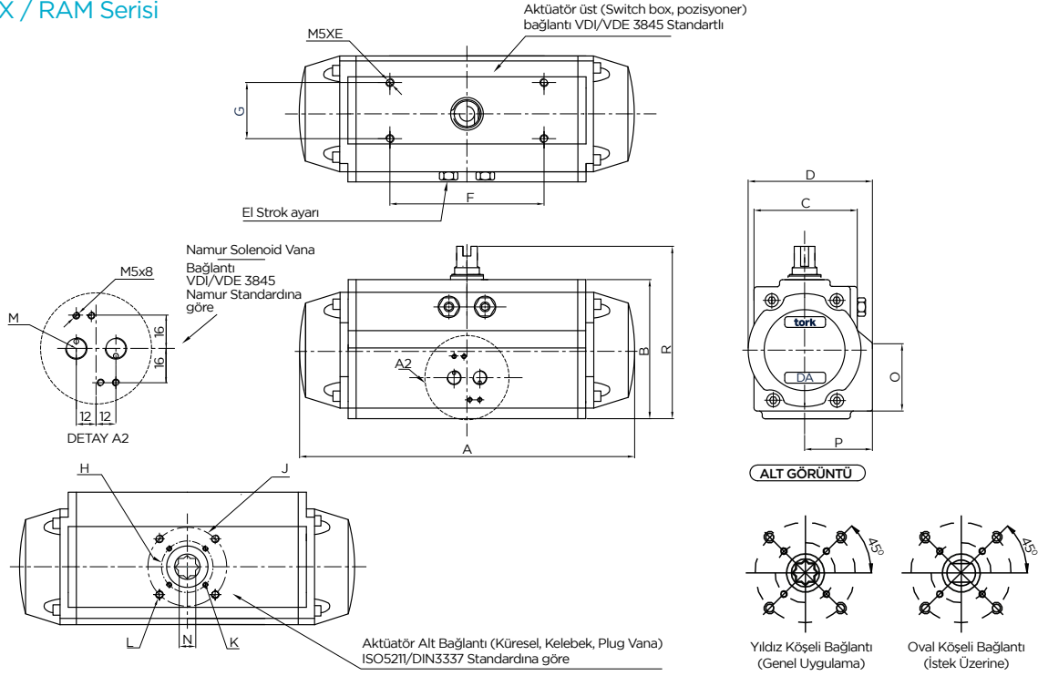
ÖLÇÜLER (mm)
